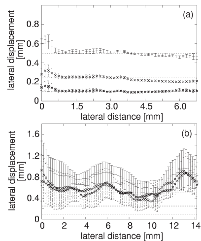
図. 模擬血管のラテラル方向変位の推定結果. プロットおよび縦棒は平均値と標準偏差を, 点線は自動ステージに与えた真値を示す. (a) 提案法. (b) 従来の位相を用いたラテラル変位推定法 (Jensen, et al.: IEEE Trans UFFC, 1998).
